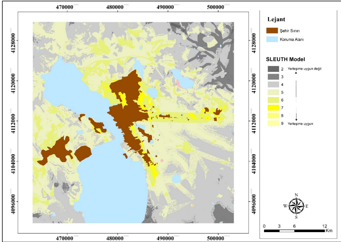
Şekil 2: AHP analizine göre oluşturulmuş SLEUTH Model
