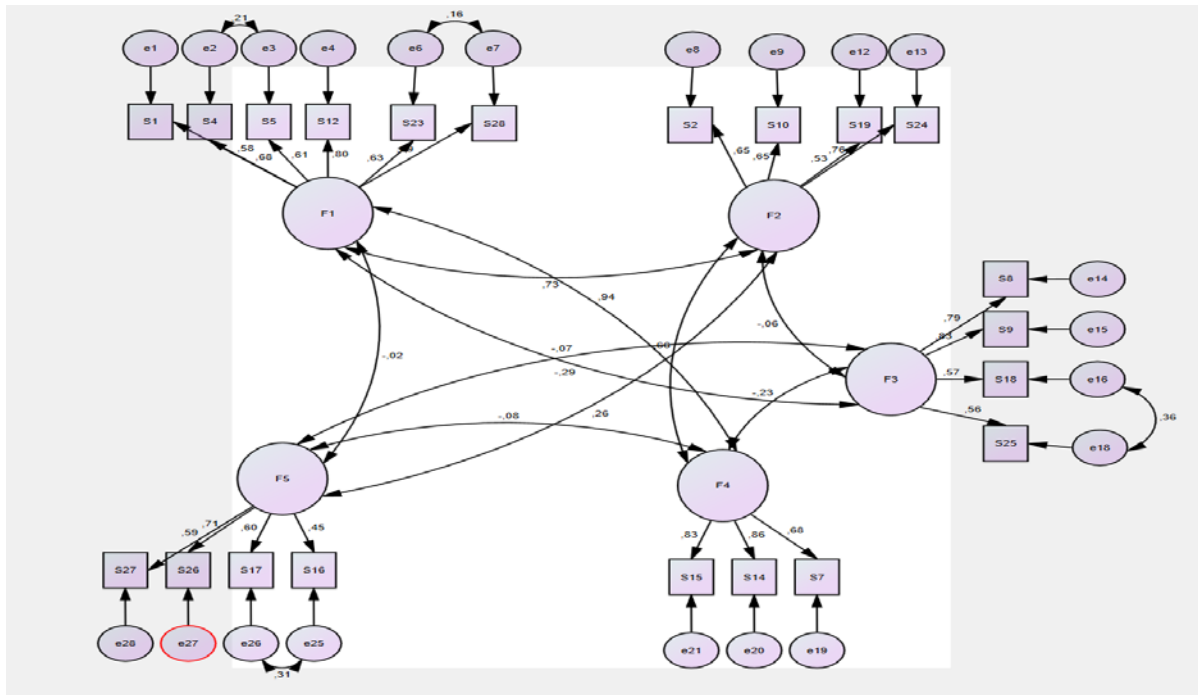
Şekil 1. Örgütsel çatışma ölçeği dfa modeli
