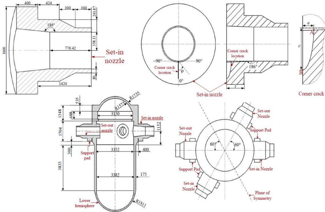
Şekil 1. RPV ve montaj nozulunun kesit görünümü [9]
