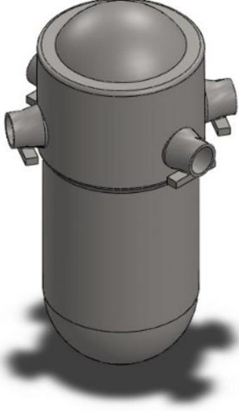
Şekil 2. Reaktör kabının montajlı katı modeli
