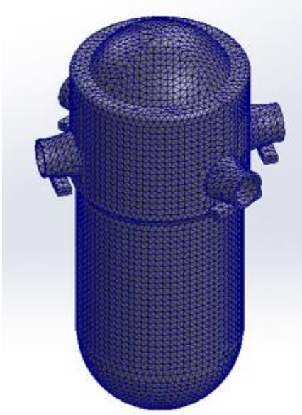
Şekil 3. Reaktör kabının mesh ağ örgüsü
