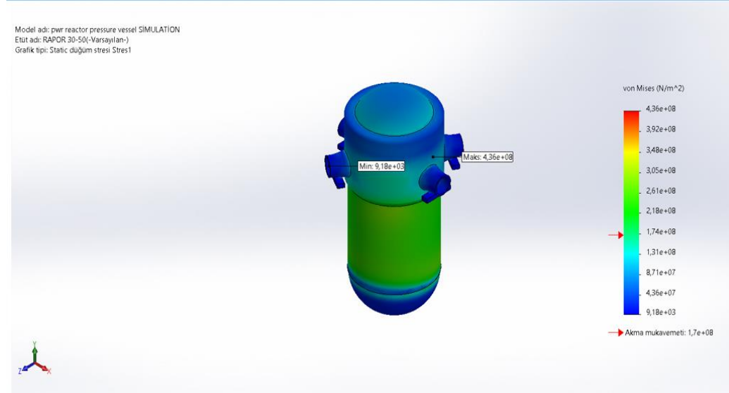
Şekil 8. AISI 316L modelin statik von mises gerilim simülasyonu
