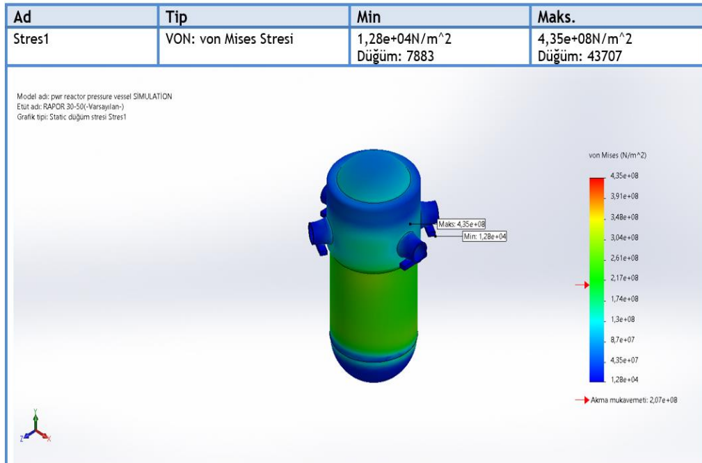
Şekil 6. AISI 304 modelin statik von mises gerilim simülasyonu
