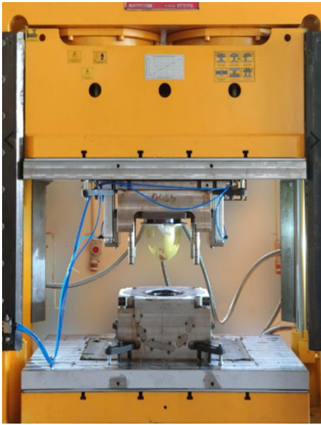
Şekil 5. Balistik Zırh Malzemesi Üretiminde Kullanılan Bir Hidrolik Pres Makinesi (Özkoç Hidrolik Makine, 2024).
