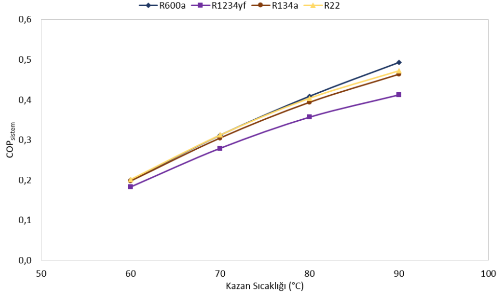
Şekil 5. Sistemin COP değerinin kazan sıcaklığı ile değişimi
