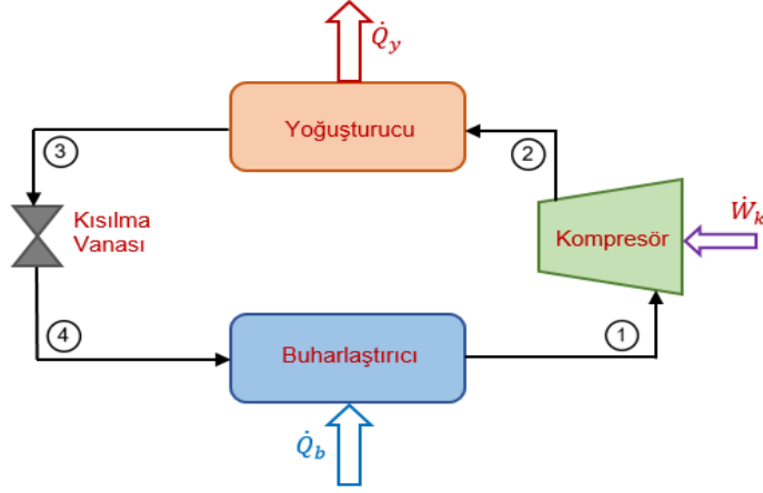
Şekil 2. Buhar sıkıştırımlı soğutma çevriminin şematik gösterimi
