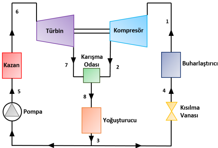
Şekil 3. Organik Rankine Çevrimi İle Birlikte Çalışan Buhar Sıkıştırma Soğutma Çevriminin Şematik Gösterimi
