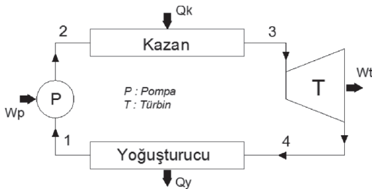
Şekil 1. Organik Rankine çevriminin şematik gösterimi
