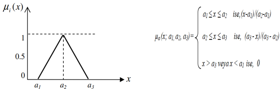
Şekil 2. Üçgen Üyelik Fonksiyonu ve Matematiksel Denklemi
