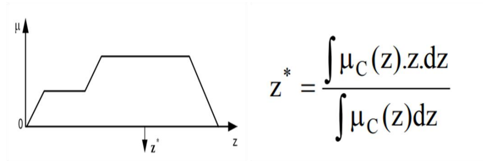
Şekil 5. Ağırlık Merkezi Yöntemi Matematiksel Denklemi ve Grafiği
