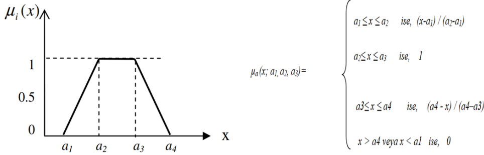
Şekil 3. Yamuk Üyelik Fonksiyonu ve Matematiksel Denklemi
