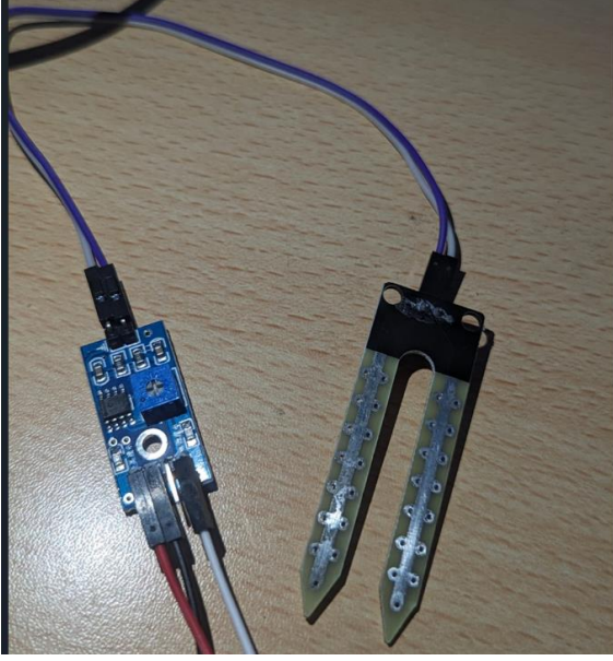
Şekil 7. Toprak nem ölçümü cihazı.
