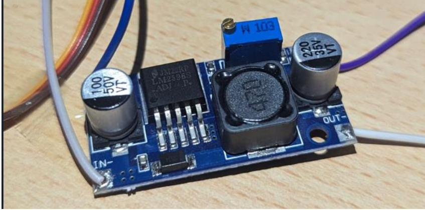
Şekil 6. 12 V-5 V Buck dönüştürücü
