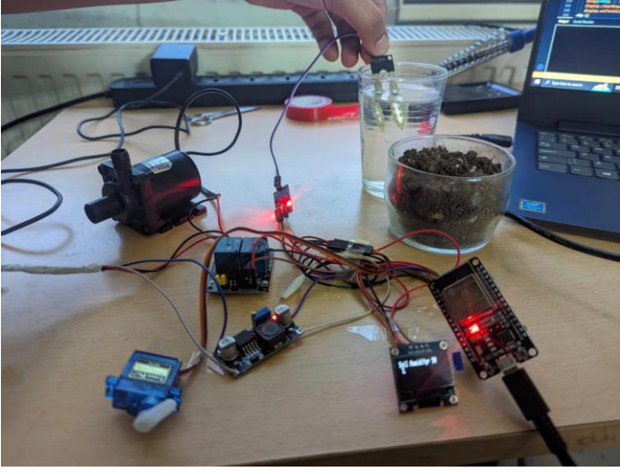
Şekil 1. Sera prototipi.
