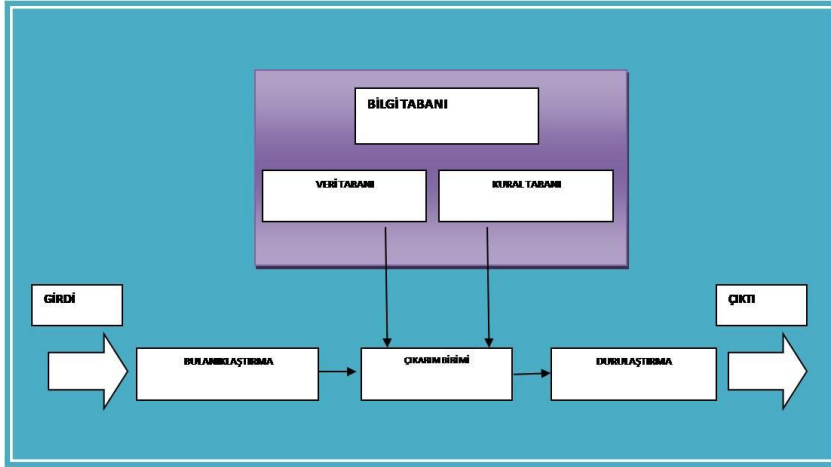
Şekil 1. Bulanık Mantık Çıkarımı
