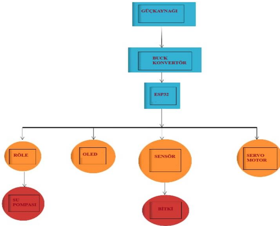
Şekil 10. Kontrol mantığı.
