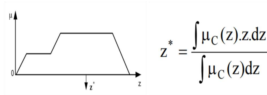
Şekil 5. Ağırlık Merkezi Yöntemi Matematiksel Denklemini ve Grafiğini
