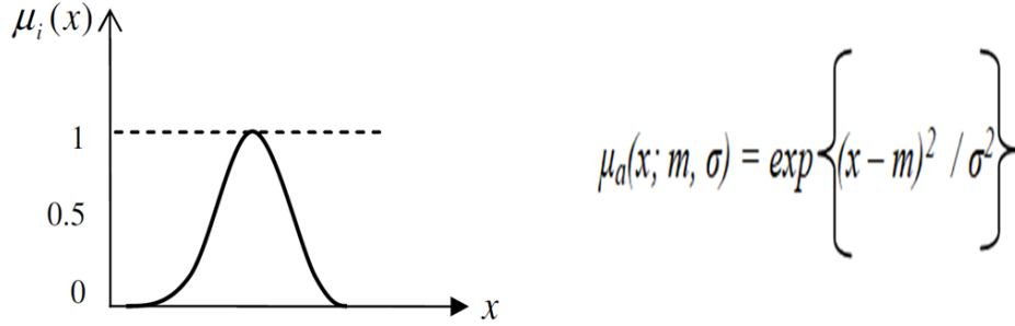
Şekil 4. Gaussian Üyelik Fonksiyonu ve Matematiksel Denklemi
