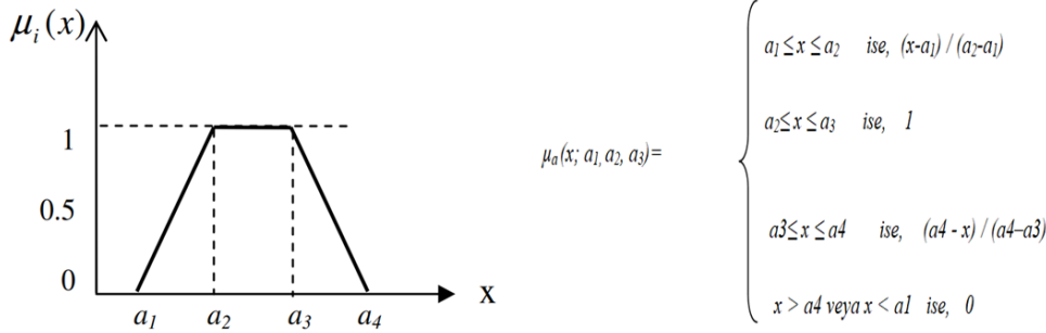
Şekil 3. Yamuk Üyelik Fonksiyonu ve Matematiksel Denklemi
